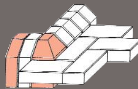
Hochbord HF 9002 Eckausbildung HF 9060
