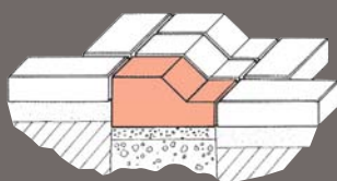
Schrägbord HF 9501
