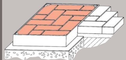
Schachtabdeckung mit Pflasterklinker ausgelegt
