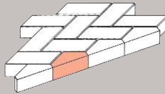
HF 9530 Endklinker für Fischgrätverlegung (Bischofsmütze)
